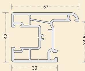
AW-1101 : S/W SASH
