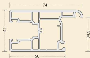
AW-1102 : S/W SUPER SASH
