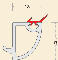
AW-1103 : S/W BEAD
