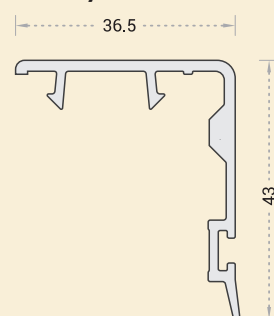
AW-1305 : S/D INTERLOCK
