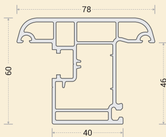
AW-2101 : C/W - SASH
