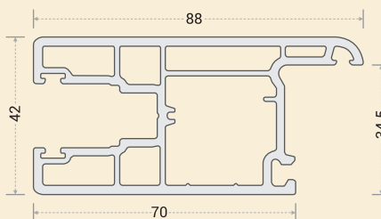
AW-1103 : S/D SASH
