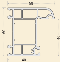
AW-2001 : C/W OF
