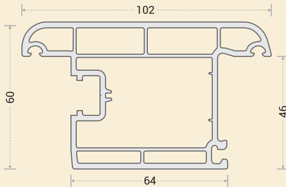
AW-2102 : C/D-T SASH
