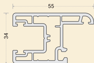
AW-1104 : S/W SASH(55)
