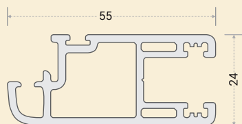
AW-1204 : S/W MESH
