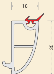
AW-2201 : CW BEAD
